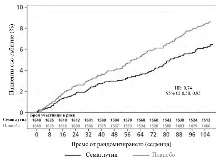
Фигура 5: Криви на Kaplan-Meier за времето до първата поява на съставния резултат: сърдечносъдова смърт, нефатален миокарден инфаркт или нефатален инсулт (SUSTAIN 6)
